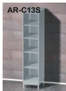
AR-C13S Шкаф на ножках 100 мм, без дверей, с 4 полками, вес 70 кг Размеры: 2000×600×500 мм цвет 7035 235,—
