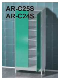
AR-C25S AR-C24S Двухдверный шкаф на ножках 100 мм, с 4 полками и замком AR-C25S Размеры: 2000×1000×500 мм цвет 7035 362,— AR-C24S Размеры: 2000×1000×400 мм цвет 7035 350,—
